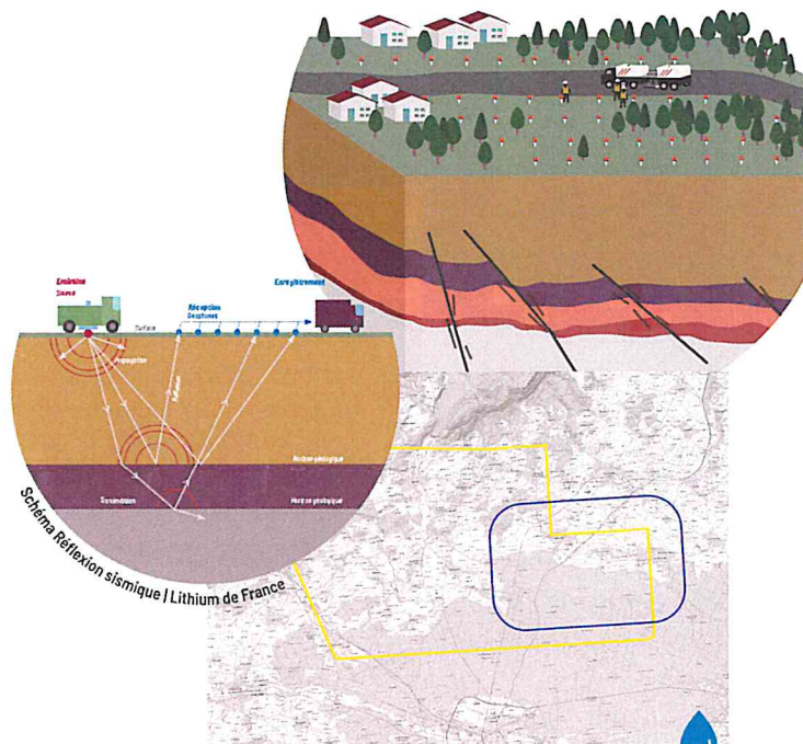
En bleu, la zone de la campagne d'exploration dans le cadre du PER «Les Sources», en jaune.
